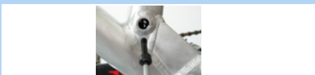
150. ábra: Postpin tengely meglazítása
