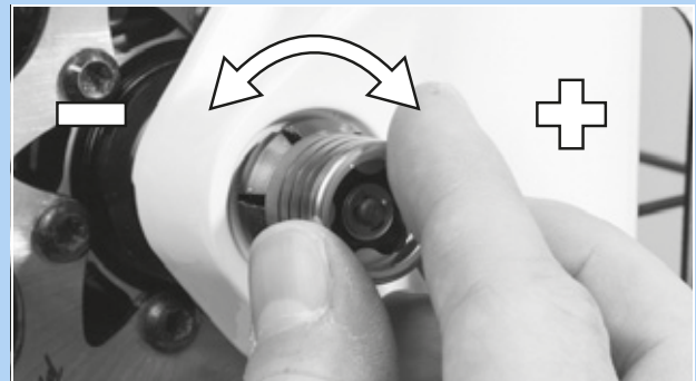
65. ábra: A feszítés beállítása
