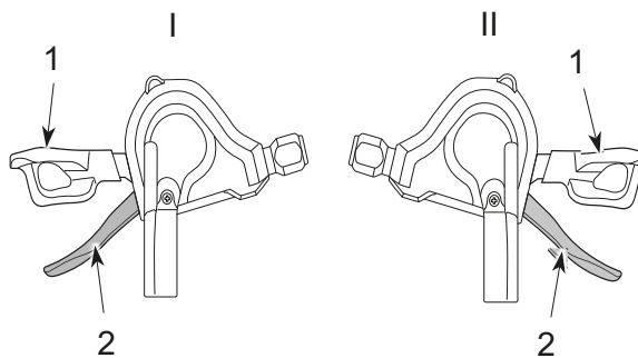
125. ábra: A bal (I) és a jobb (II) váltó lekapcsoló karja (1) és felkapcsoló karja (2)
